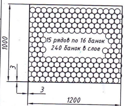
Схема упаковки банок в палете
